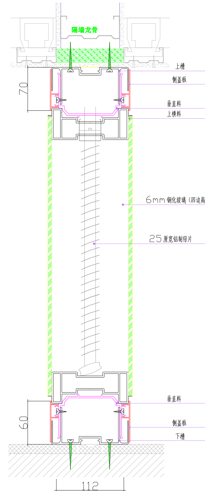
剖面图 (玻璃+百叶帘)
